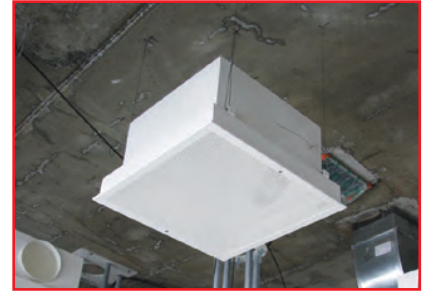
Plenum boxes
